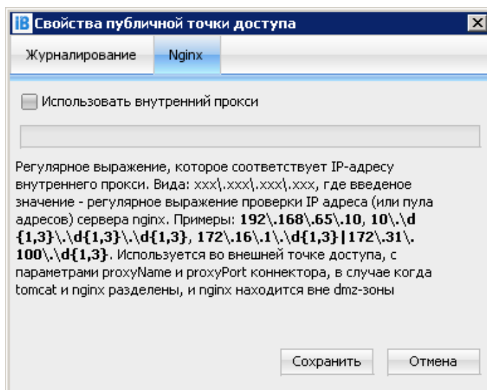
Рис. 19. Окно "Свойства публичной точки доступа". Закладка "Nginx"
